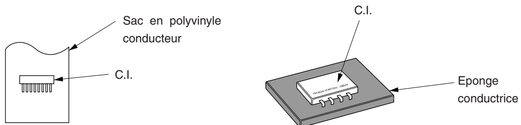
Fig. 1 Emballage conducteur
