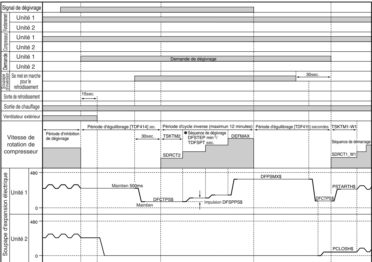
• Diagramme des temps pendant l'exécution du dégivrage (uniquement l'unité 1 en fonction, l'unité 2 arrêtée)
