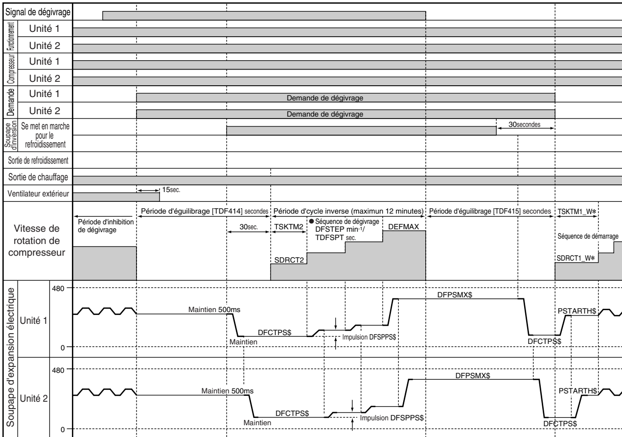
• Diagramme des temps pendant l'exécution du dégivrage (les deux unité 1 et unité 2 en fonction)
